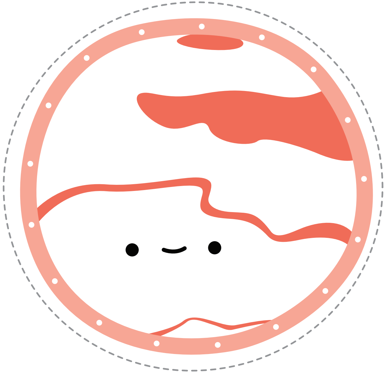
mars
