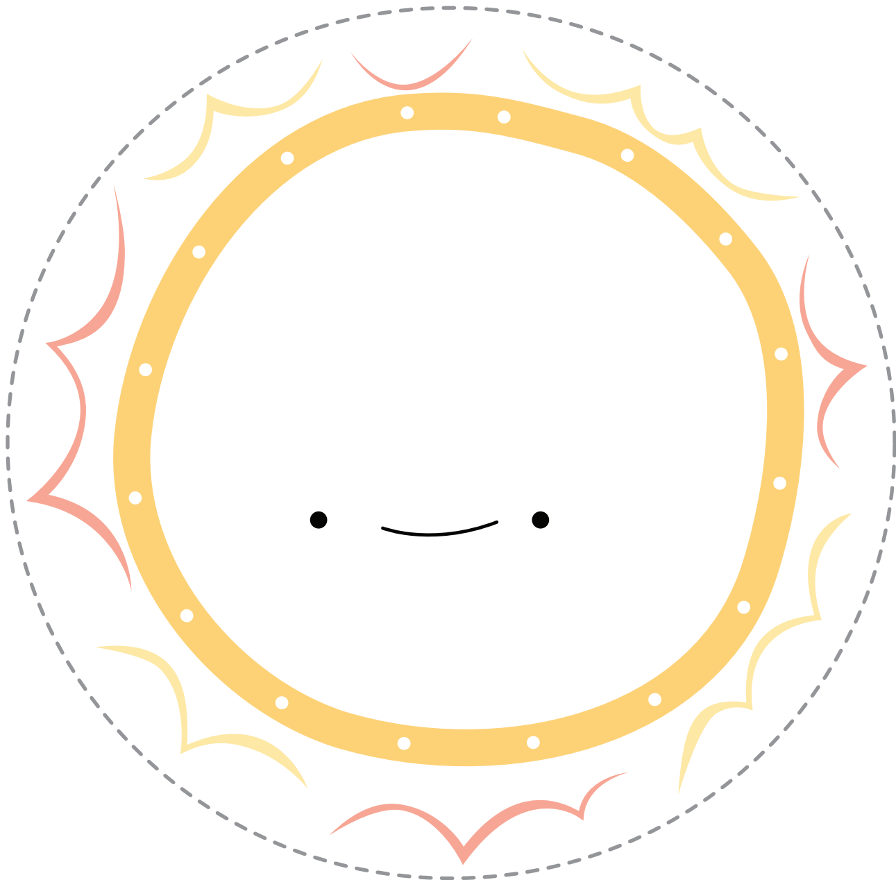
sun
